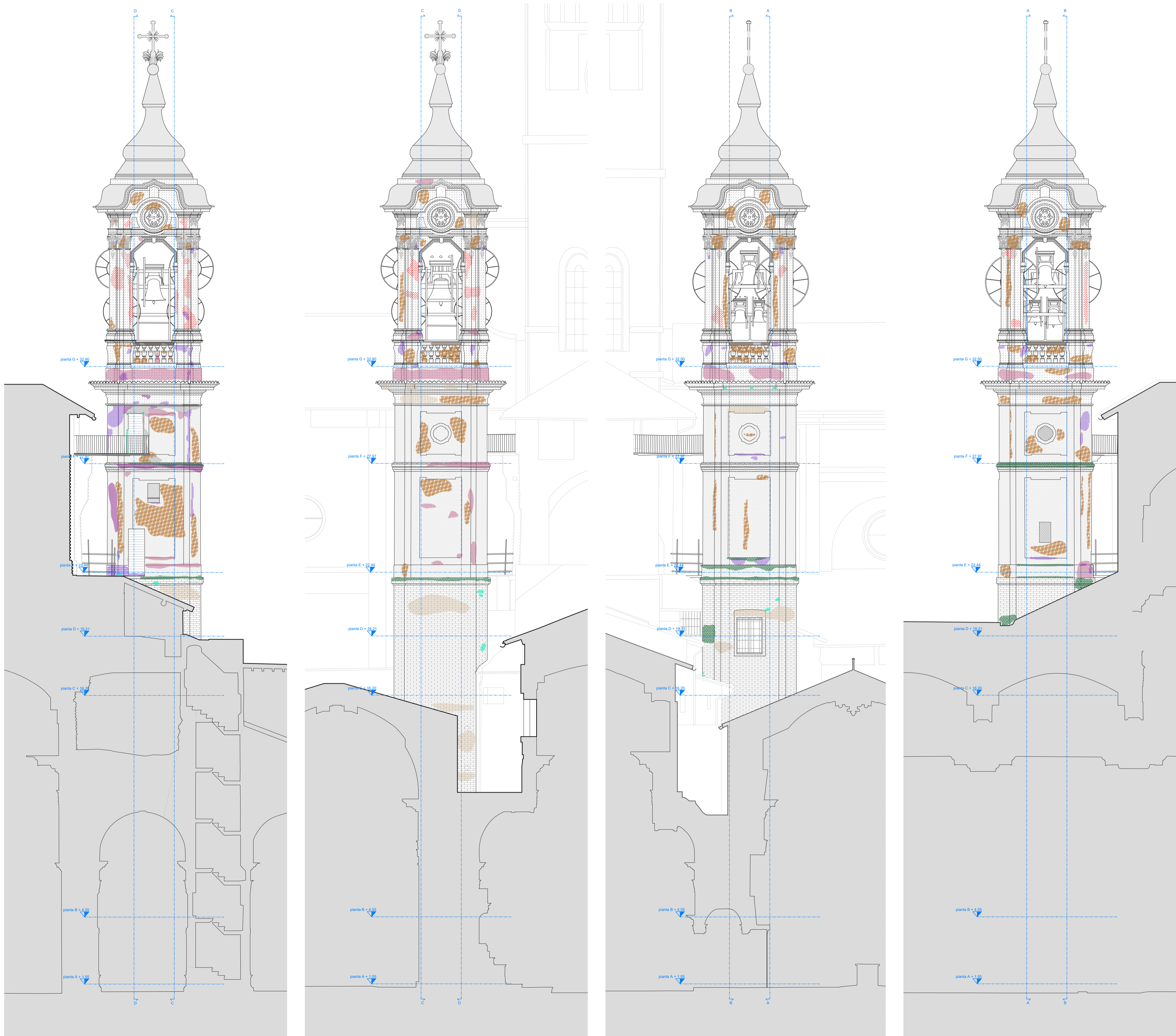
01 STATO DI FATTO - PROSPETTO SUD 1:100 02 STATO DI FATTO - PROSPETTO NORD 1:100 03 STATO DI FATTO - PROSPETTO EST 1:100 04 STATO DI FATTO - PROSPETTO OVEST 1:100
