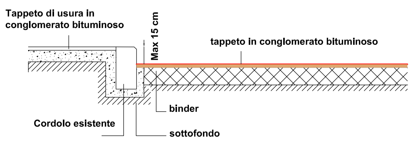
SEZIONE TIPO - scala 1:20
