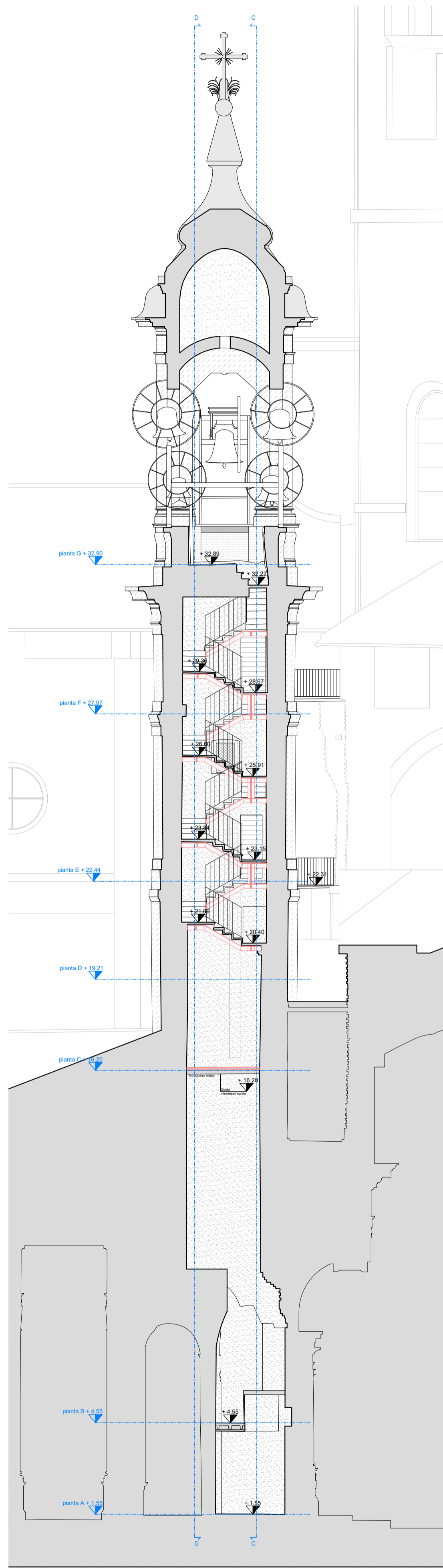
01 CONFRONTI - SEZIONE A-A' 1:100
