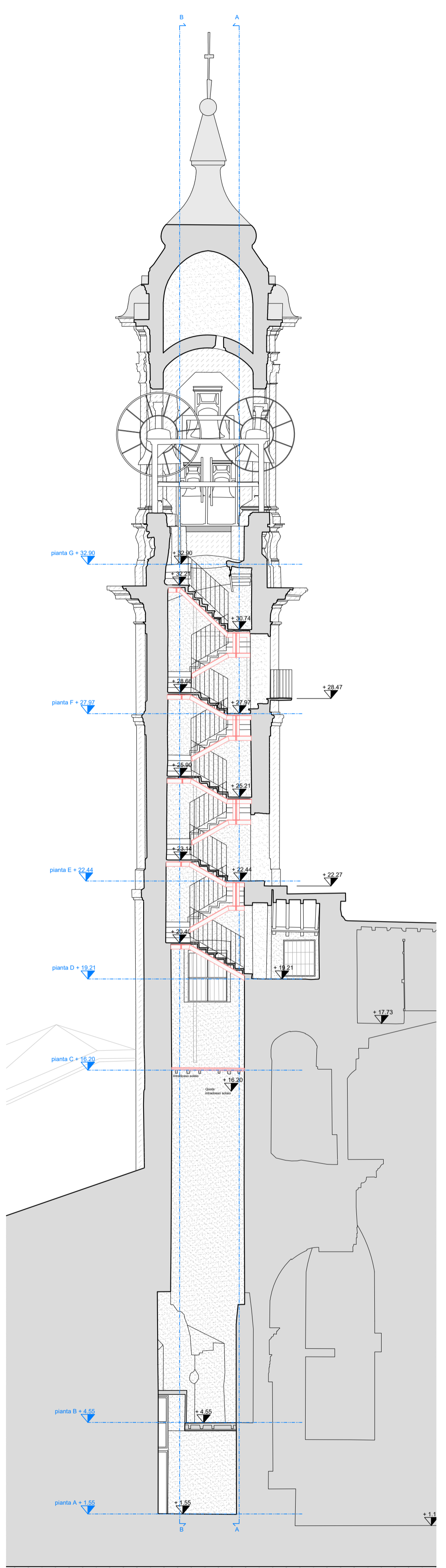
03 CONFRONTI - SEZIONE C-C' 1:100
