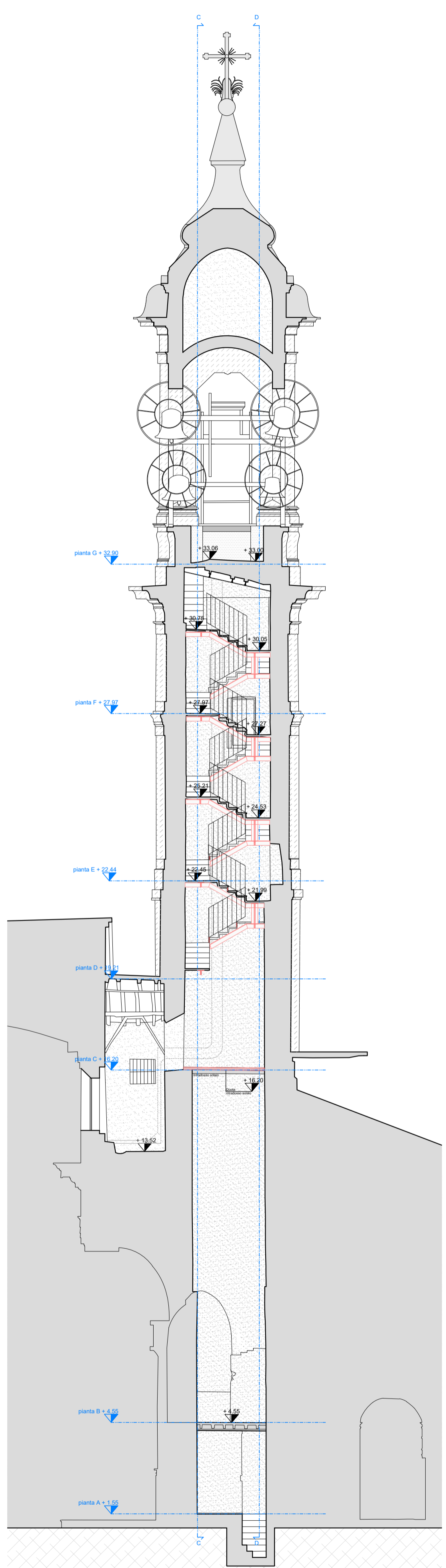
02 CONFRONTI - SEZIONE B-B' 1:100
