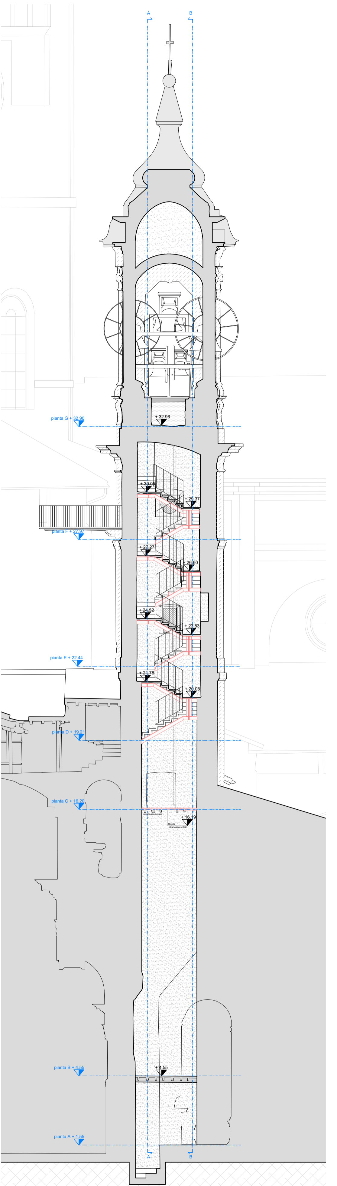
04 CONFRONTI - SEZIONE D-D' 1:100
